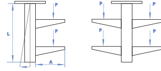
U DESTEK STATİK DEĞERLERİ U SUPPORT STATIC VALUES
